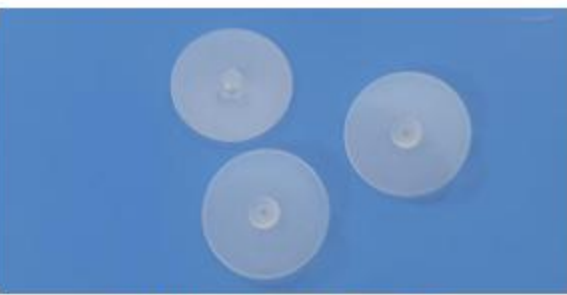
S1500伞形直径：29mm 阀杆直径：3.6mm 扣柱高度：2.1mm
