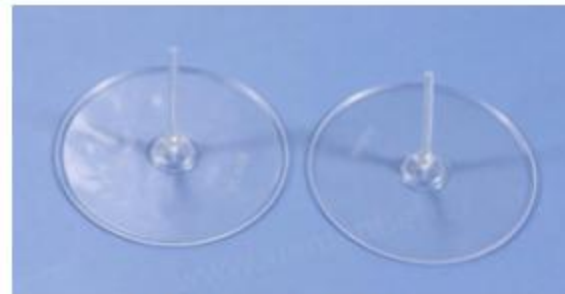
S407伞形直径：36mm 阀杆直径：1.7mm 扣柱高度：1.5mm
