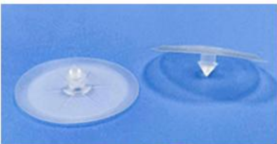
S1694伞形直径：30mm 阀杆直径：3.7mm 扣柱高度：2.5mm
