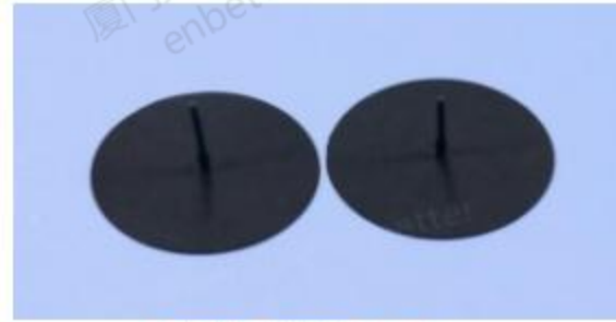
S1251伞形直径：24mm 阀杆直径：1mm 扣柱高度：1.5mm
