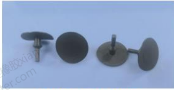
S0219伞形直径：18mm 阀杆直径：3.8mm 扣柱高度：4.5mm 伞面厚度：0.6~0.7mm
